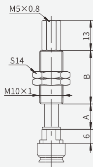
Suction cup 3.5×7 4×10 5×10 6×10
