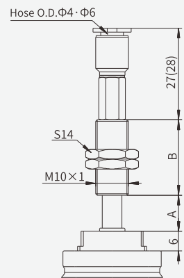
Suction cup 4×30 5×30 6×30 8×30
