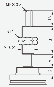
Suction cup 4×30 5×30 6×30 8×30
